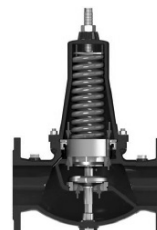
Клапан полностью закрыт (нет разбора).
